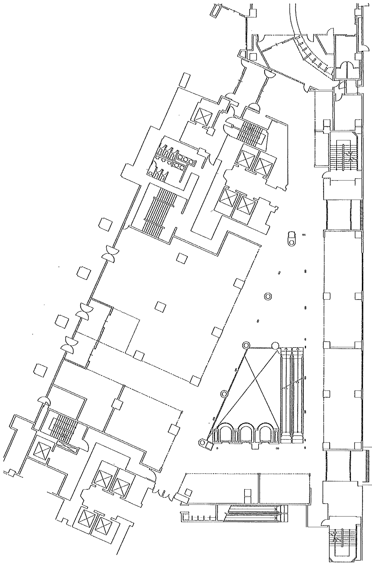
1 階平面図
